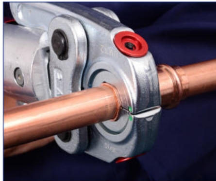
5. Fertigstellung der Verbindung mithilfe des Presswerkzeugs
