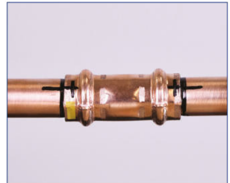
6. Verpresste Verbindung markieren
