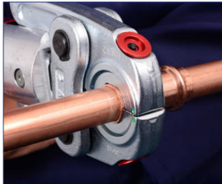
5. Fertigstellung der Verbindung mithilfe des Presswerkzeugs
