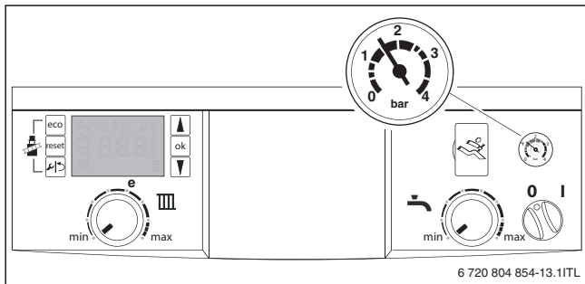
Bild 4 Manometer zur Kontrolle des Betriebsdrucks bei geöffneter Bedienblende
