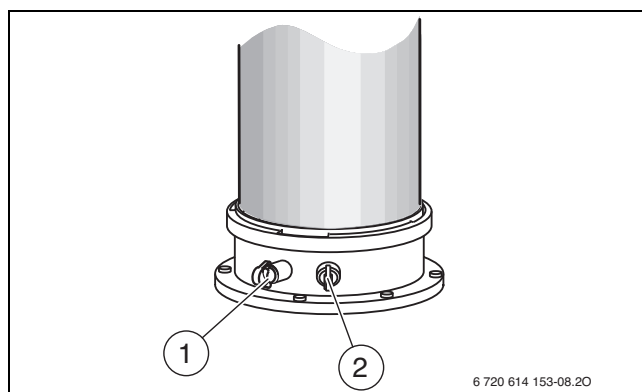
Bild 55 Abgassonde und Verbrennungsluft-Messstutzen
