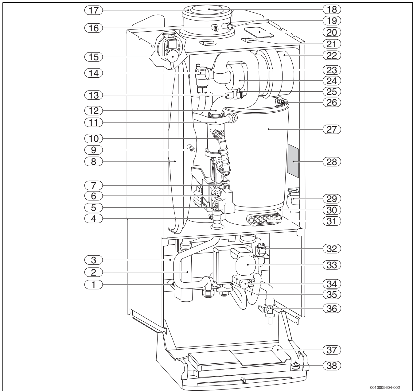
Bild 3 Produktübersicht
