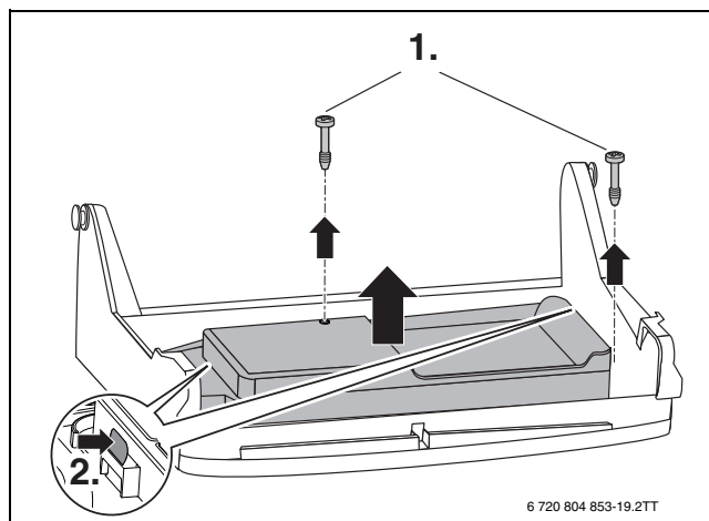
Bild 79 Abdeckung entfernen
