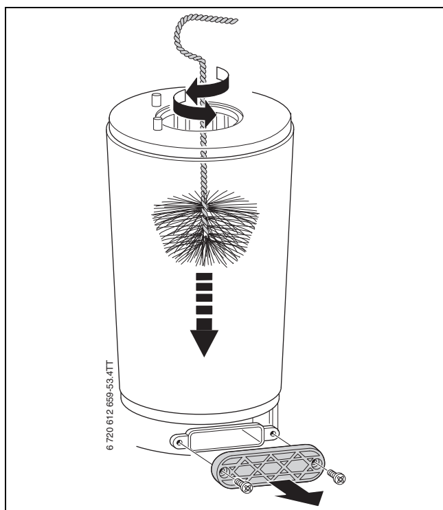
Bild 62 Wärmeblock reinigen
