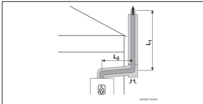
Bild 14 Konzentrische Luft-Abgas-Führung nach C_{53x} an der Außenwand
