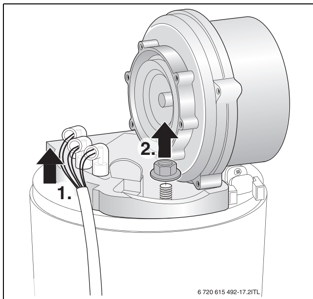
Bild 58 Gebläse herausnehmen
