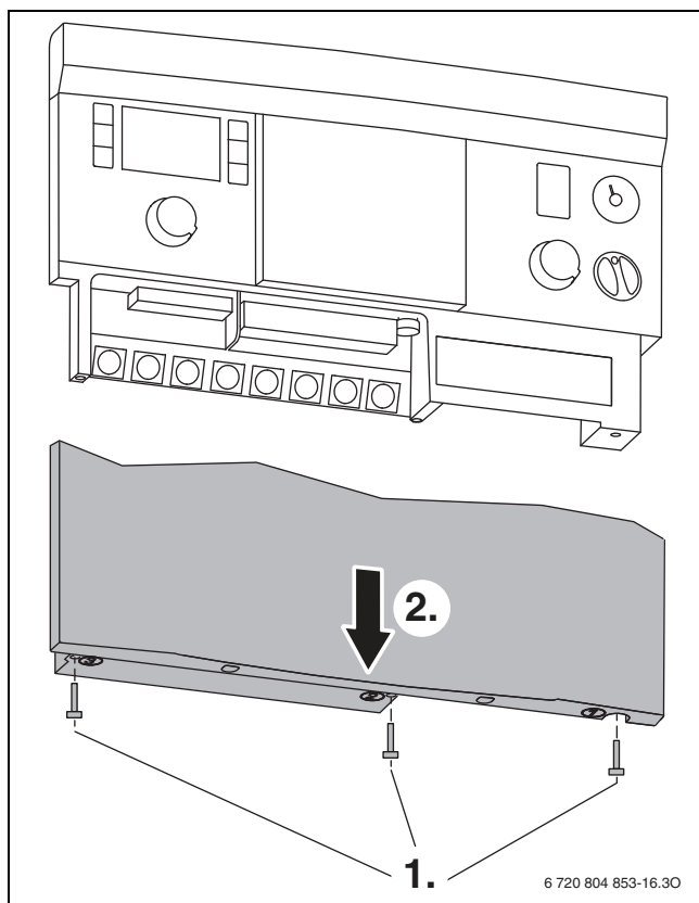
Bild 77 Abdeckung entfernen
