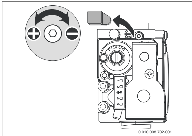
Bild 49 Plombe entfernen
