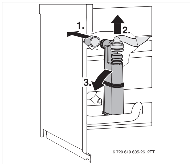
Bild 65 Kondensatsiphon ausbauen
