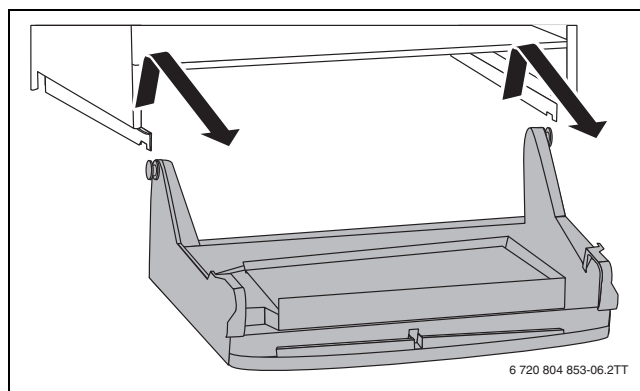
Bild 80 Steuergerät aushängen
