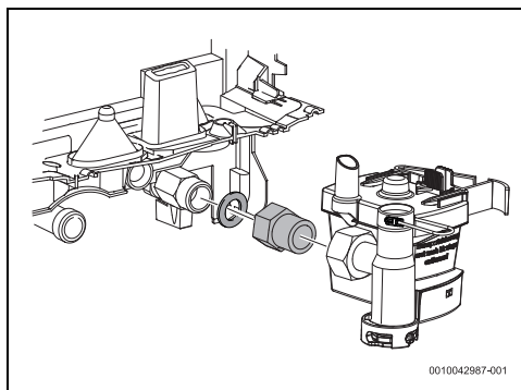
Fig. 27 Bague supplémentaire
