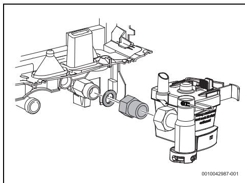
Bild 28 Zusätzliche Buchse
