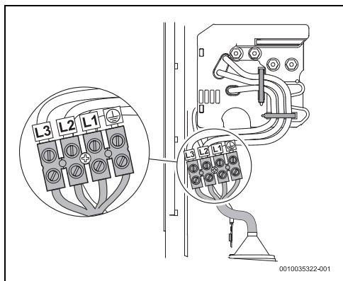
Bild 43 Anschluss unten
