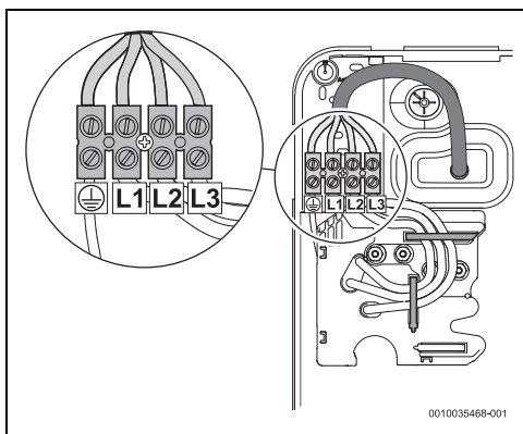
Fig. 41 Raccord supérieur
