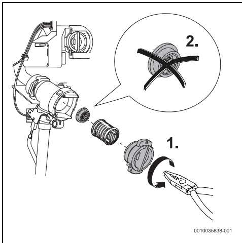
Bild 56 Durchflussbegrenzer entfernen.
