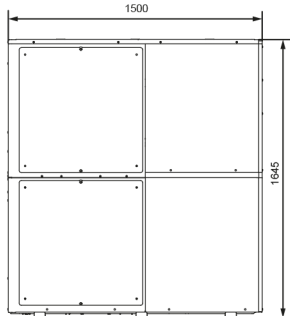
Frontansicht
