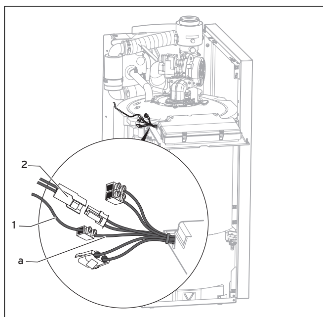
Abb. 5.5 Speicherfühler und Ladetemperaturfühler anschließen (actoSTOR)
