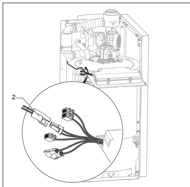
Abb. 5.6 Speichertemperaturfühler anschließen
