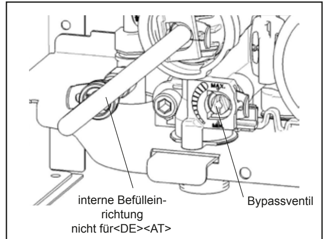
Bild: Bypassventil
