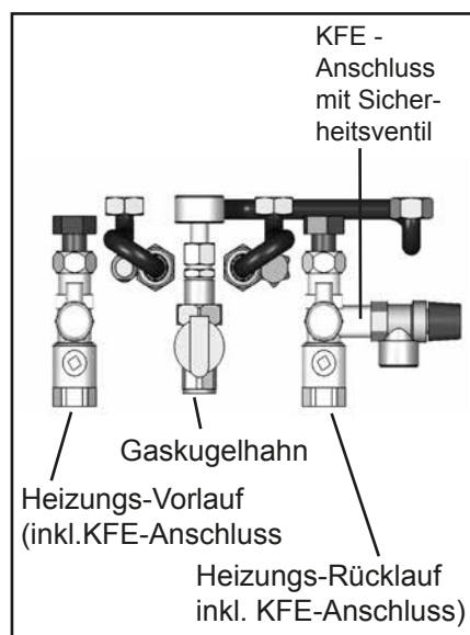
Bild: Absperrarmaturen (Zubehör)
