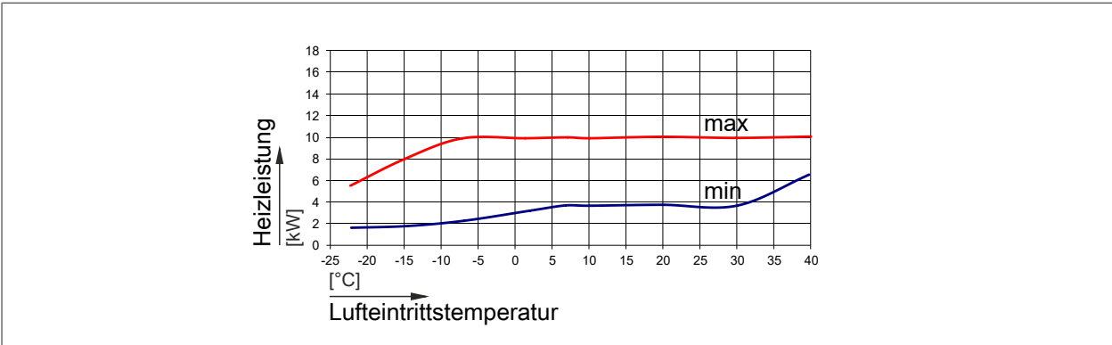
Abb. 10: Heizleistung CHA-10 bei einem Vorlauf von 25 °C
