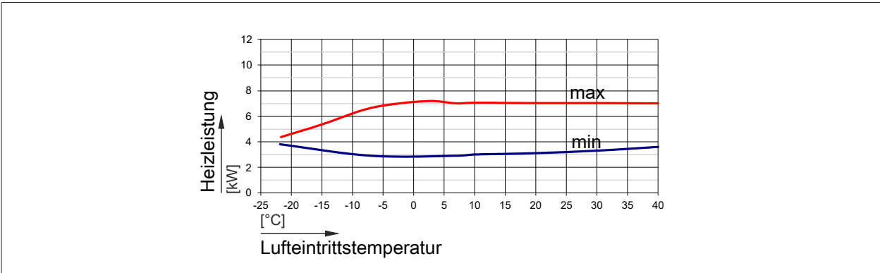
Abb. 7: Heizleistung CHA-07 bei einem Vorlauf von 45 °C
