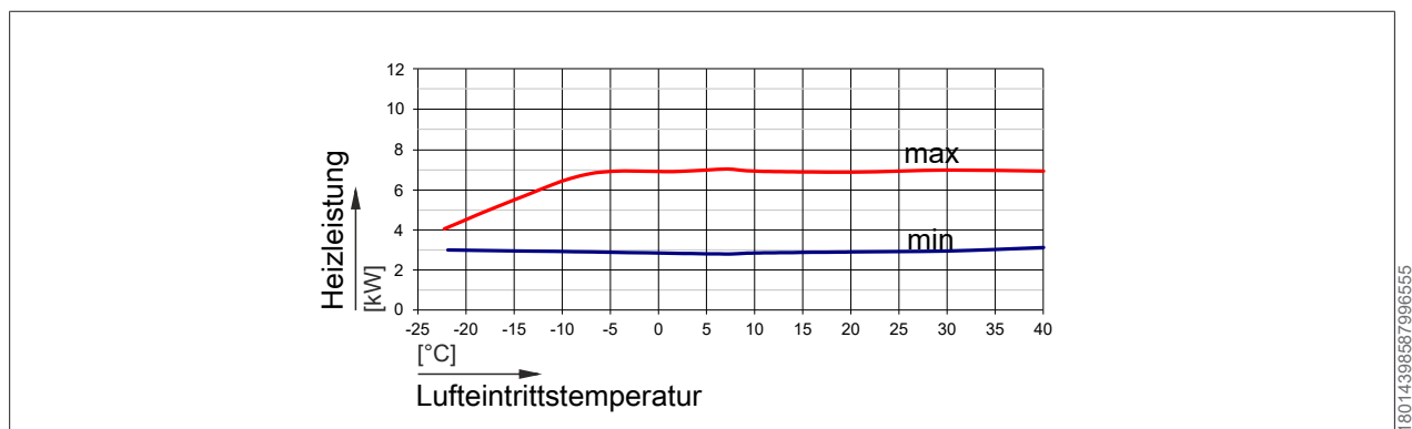
Abb. 6: Heizleistung CHA-07 bei einem Vorlauf von 35 °C
