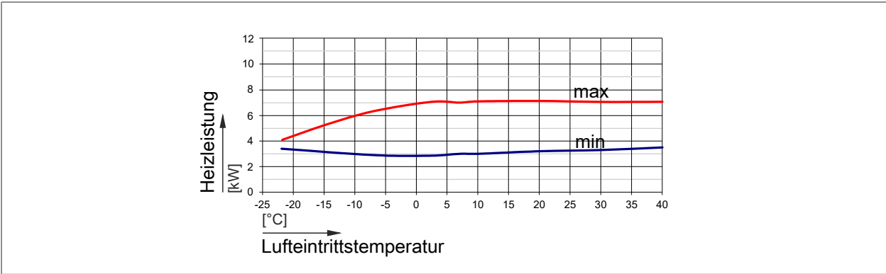
Abb. 8: Heizleistung CHA-07 bei einem Vorlauf von 55 °C
