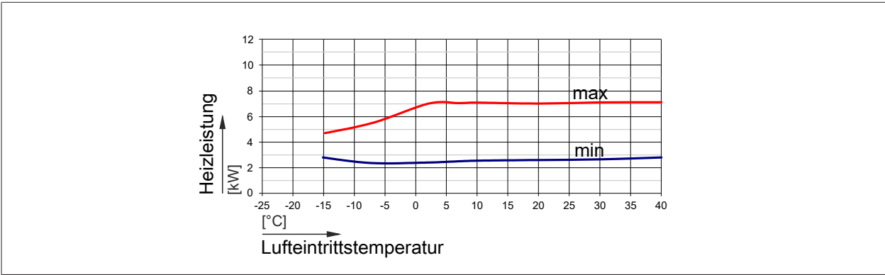
Abb. 9: Heizleistung CHA-07 bei einem Vorlauf von 65 °C
