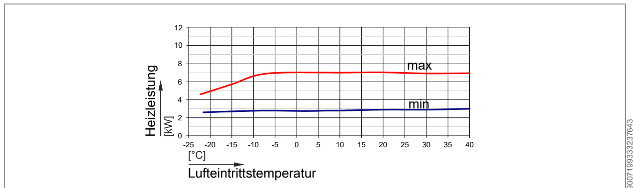
Abb. 5: Heizleistung CHA-07 bei einem Vorlauf von 25 °C
