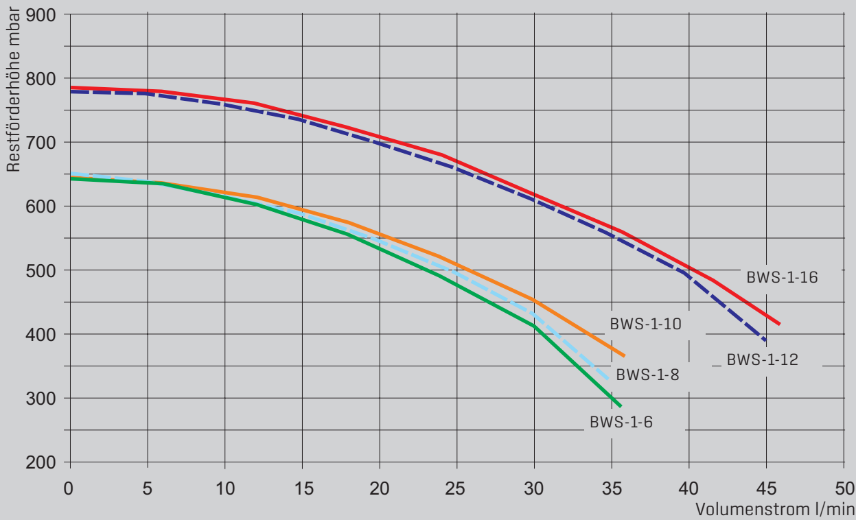
RESTFÖRDERHÖHE HEIZKREIS BWS-1-06 BIS BWS-1-16
