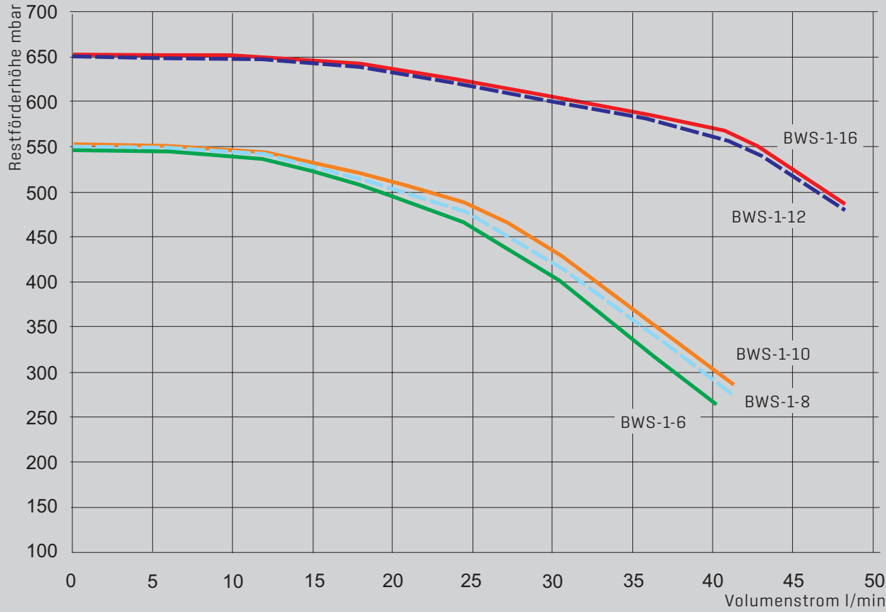
RESTFÖRDERHÖHE SOLEKREIS BWS-1-06 BIS BWS-1-16 BEI 0°C SOLETEMPERATUR
